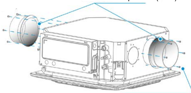
Vis de raccordement de la bride (12)
