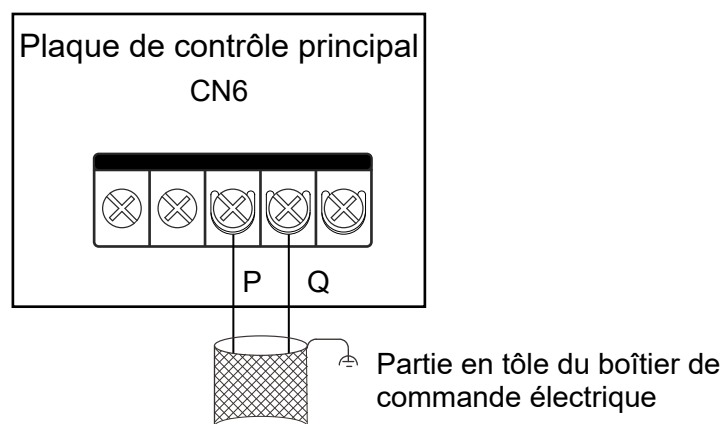
Connexion aux ports PQ de l'UE
