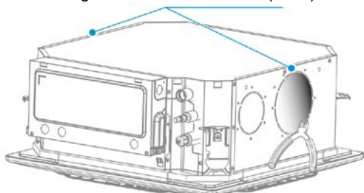
Trous de débouchage de l'unité d'extension (deux)
