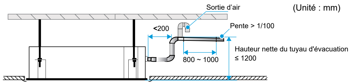
Méthode de raccordement du tuyau d'évacuation pour un seul appareil.
