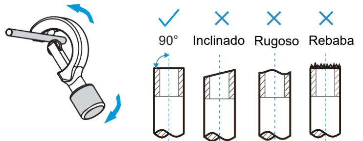
Cortatubos
