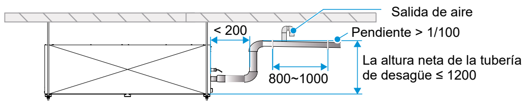
Cómo conectar el tubo de desagüe para la bomba de desagüe de una sola unidad
