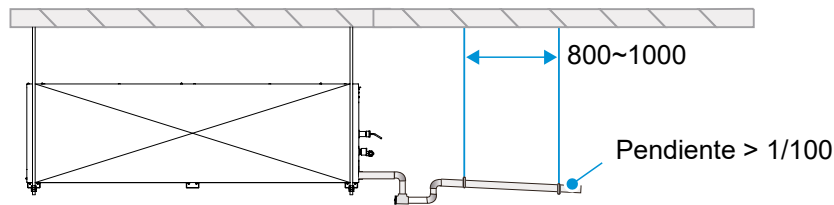
Método de conexión del tubo de desagüe para una sola unidad
