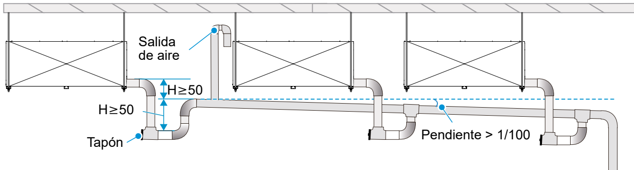
Las tuberías de desagüe de varias unidades se conectan a la tubería de desagüe principal para ser drenadas a través de la tubería de alcantarillado.
