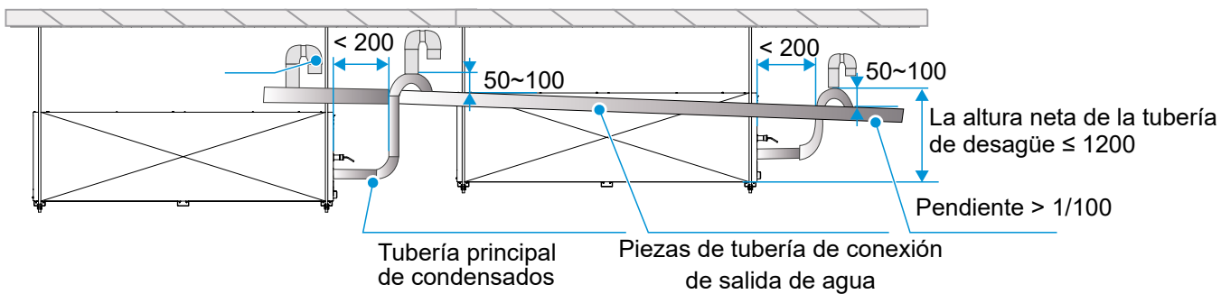
Cómo conectar el tubo de desagüe para la bomba de desagüe de una sola unidad
